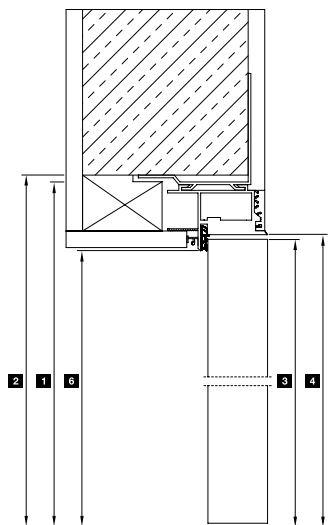
Vertikalni presjek s vratnim krilom u ravni
