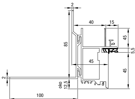
Dimenzije Zeroline dovratnika
