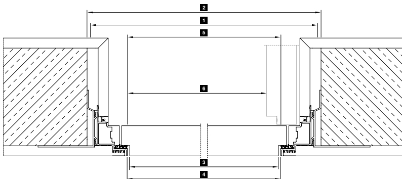
Horizontalni presjek s Reverse vratnim krilom
