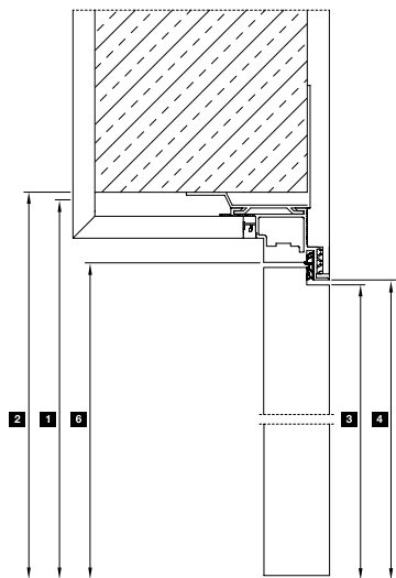
Vertikalni presjek s Reverse vratnim krilom
