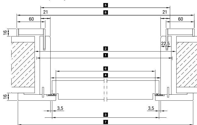
Horizontalni presjek
