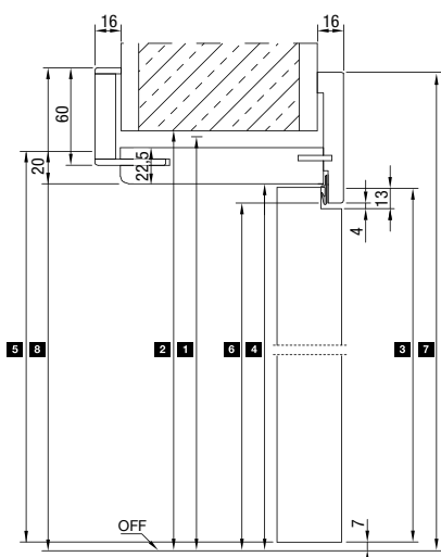
Vertikalni presjek
